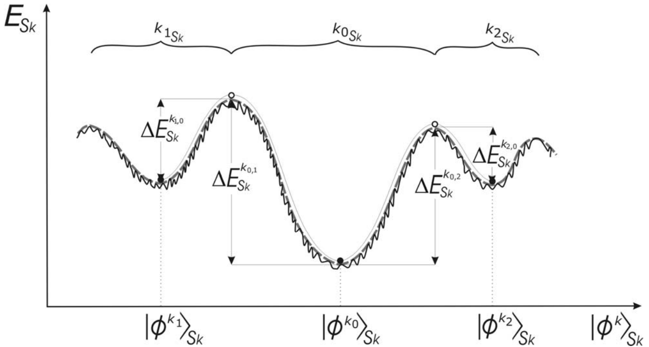
Slika 1. Šematska prezentacija memorijskih atraktora u prostoru energija-stanje ( E_{S_k}(\phi^{k_i}) ) kvantno-holografске memorije/propagatora makroskopskog otvorenog kvantnog akupunktornog sistema/svesti S_k [1,2]:
